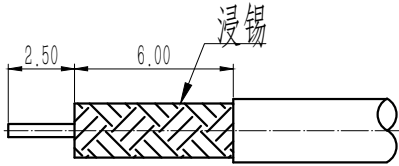
建议剥线尺寸
